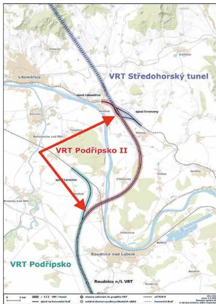
Přehled navrhovaného vedení úseku VRT Podřipsko II. v našem regionu. Zdroj: Správa železnic
